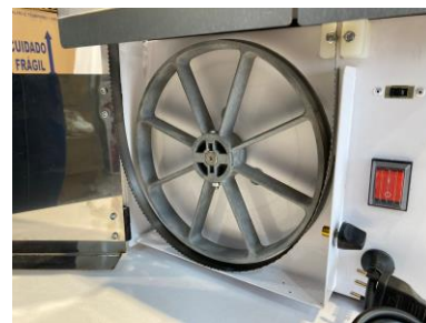
9) Encaixar a Lâmina de Corte no Volante Inferior.
