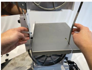
7) Acomodar a Lâmina de Corte. Nota: A Serra de Corte deverá ficar voltada para o operador.
